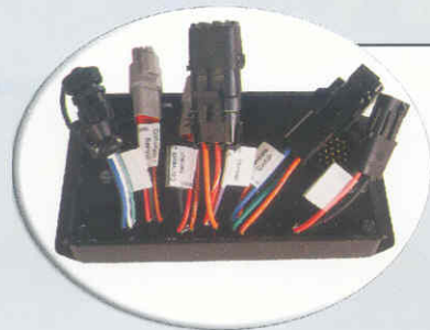
Caixa controladora - regula a abertura da válvula eletro-hidráulica.
