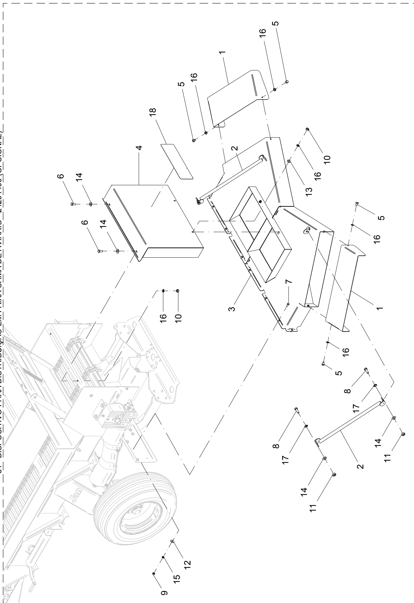
34 - DISPOSITIVO PARA DISTRIBUIÇÃO EM FAIXA CAMA DE AVIÁRIO - 24204400 (OPCIONAL)
