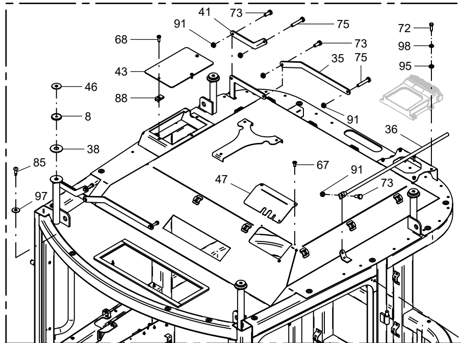
DETALHE A
