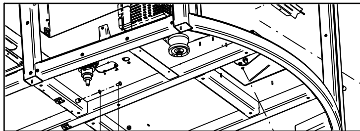
DETALHE INFERIOR
